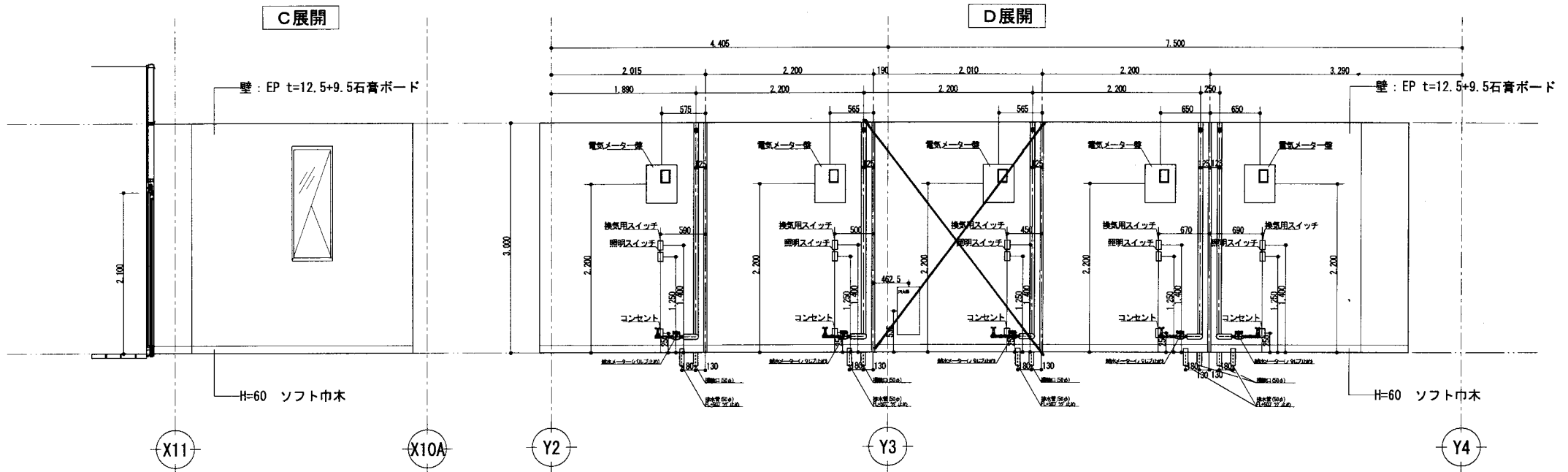
チャレンジショップ展開図 S=1/50
